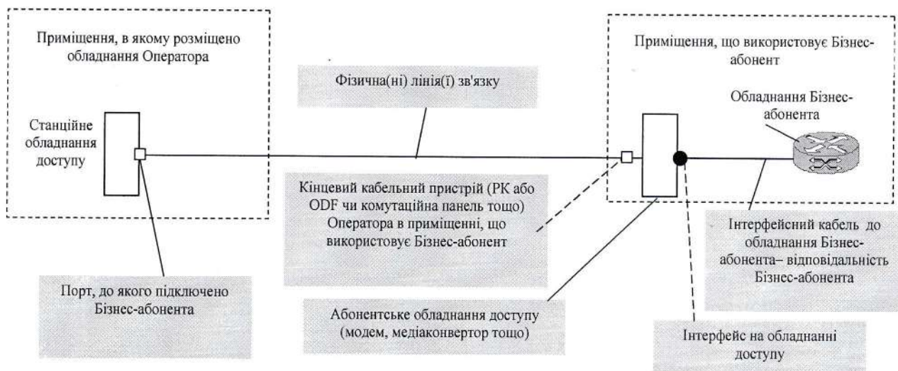
Рис. Конфігурація та схема надання Послуги «Інтернет» (зони відповідальності Сторін зазначені у Замовленні про надання/зміну Послуги «Інтернет»)
